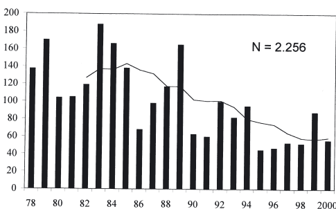
Årsfordeling af Gråmåge 1978-2000. Annual numbers of Glaucous Gull 1978-2000.
