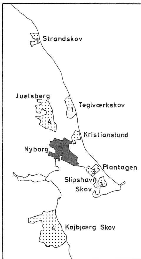
Fig. 5. Det anslåede antal ynglepar i skovene omkring Nyborg, Østfyn. Materialet baseret på RABØL (1966).
