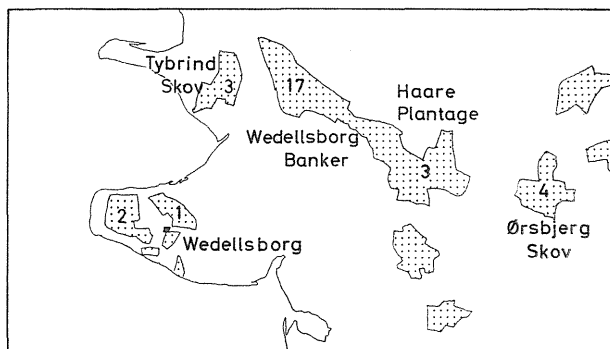
Fig. 4. Det anslåede antal ynglepar i skovene omkring Wedellsborg, Vestfyn (maj. 1962–maj. 1963).
