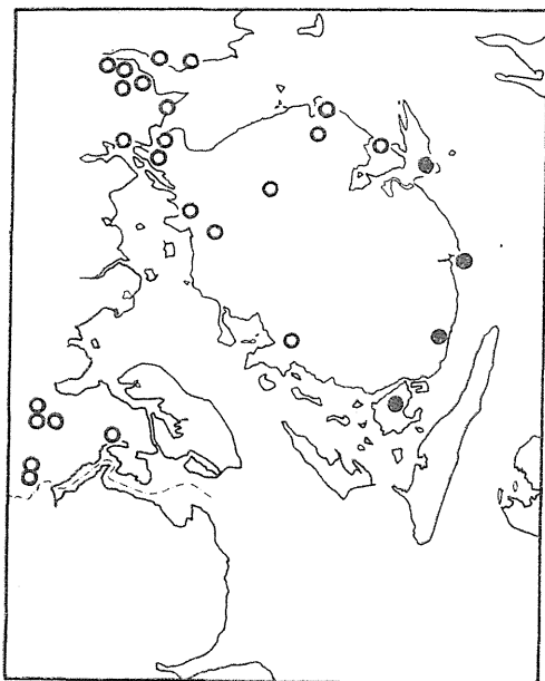
Fig. 1. Lokalteter, hvor Topmejsen er iagttaget i perioden 1943–1950. Der er ikke skelnet mellem redefund og iagttagelser uden forbindelse med redefund. De enkelte forekomster er beskrevet i appendix 1.
