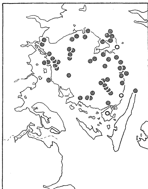
Fig. 2. Lokalteter på Fyn, hvor Topmejsen er iagttaget i perioden 1950–1967. Åbne cirkler angiver steder, hvorfra der foreligger tidligere iagttagelser, men hvor arten ikke er truffet i den nævnte periode.
