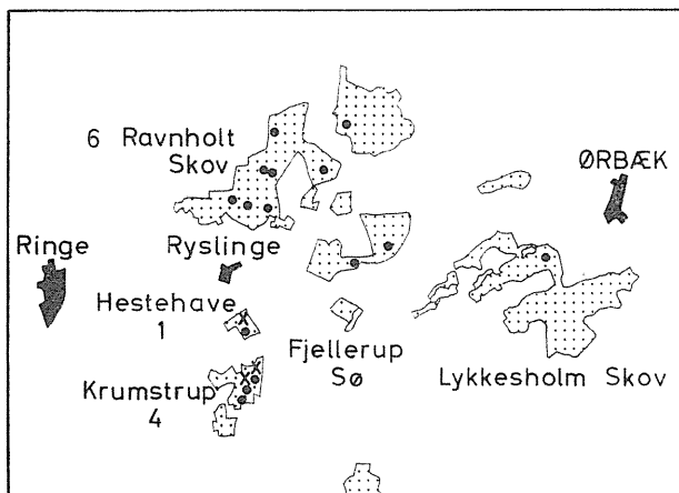
Fig. 3. Iagttagelser af Topmejsen fra hele året (i årene 1963–67) i Ravnholtskovene, Lykkesholmskovene og Ryslinge Hestehaveskov og Krumstrup på det centrale Fyn. Ynglefund er angivet med et kryds. Tallene ved tre skove angiver det anslåede antal ynglepar.
